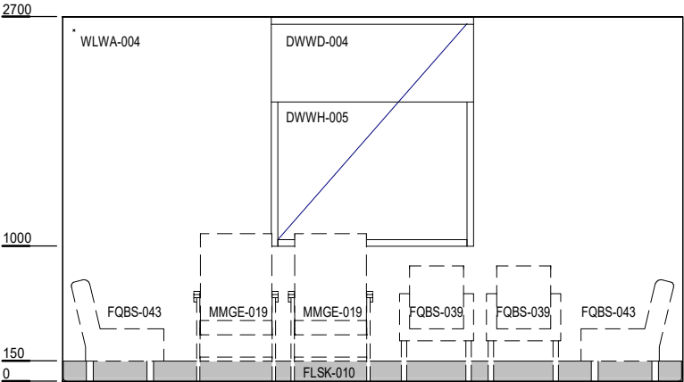
ELEVATION 1
