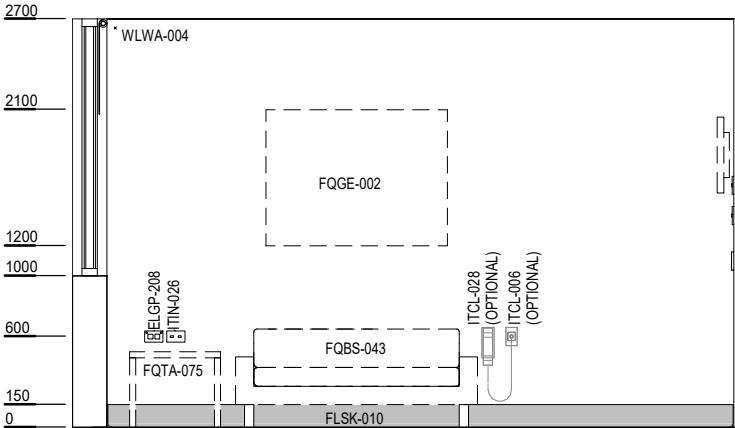
ELEVATION 2
