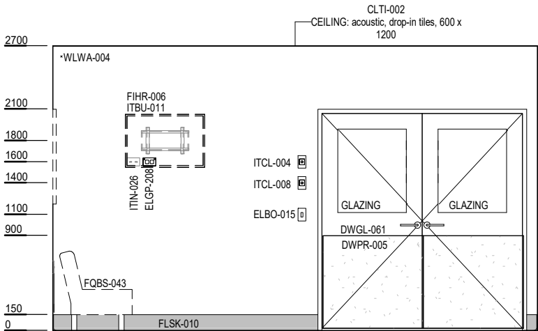
ELEVATION 3
