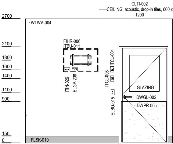
ELEVATION 3
