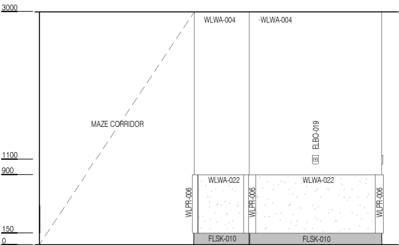
ELEVATION 6
