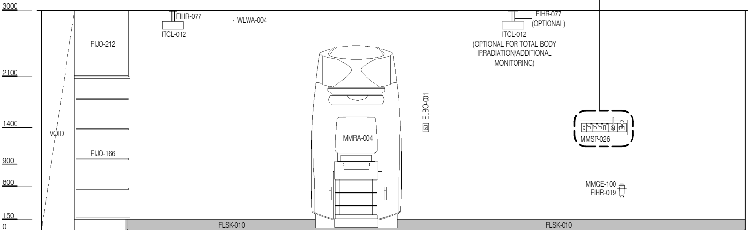
ELEVATION 4
