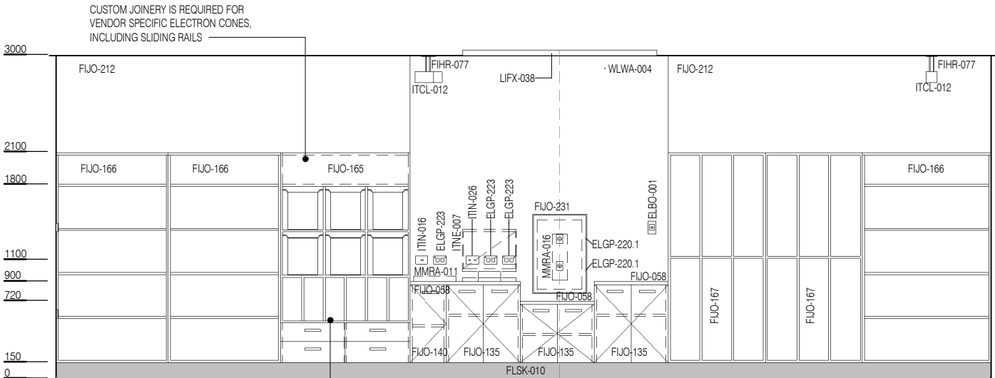
ELEVATION 3
