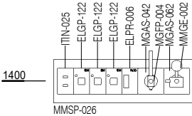
ELEVATION 11( 1 : 25 @ A3 )
