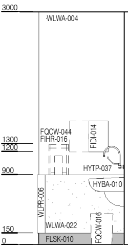
ELEVATION 5
