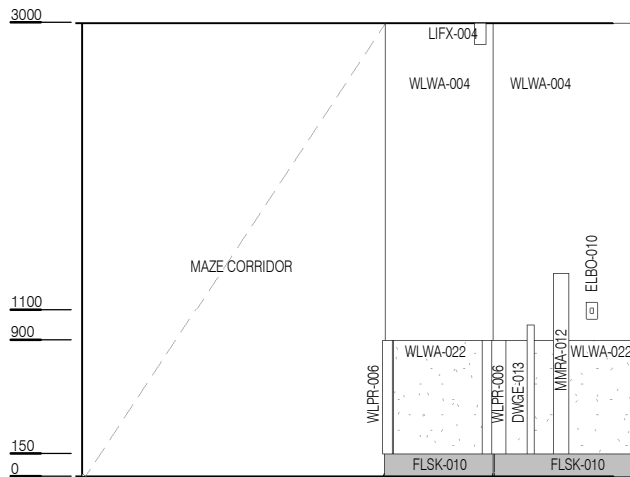
ELEVATION 7
