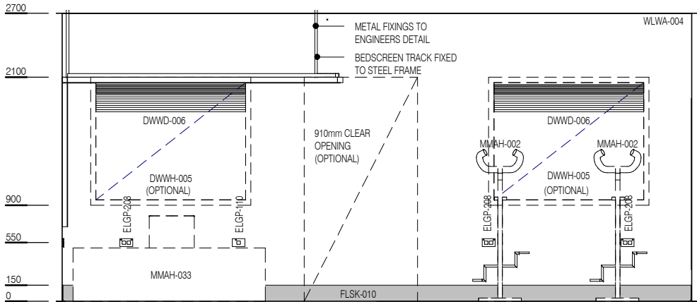
ELEVATION 1
