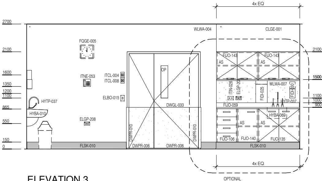
ELEVATION 3
