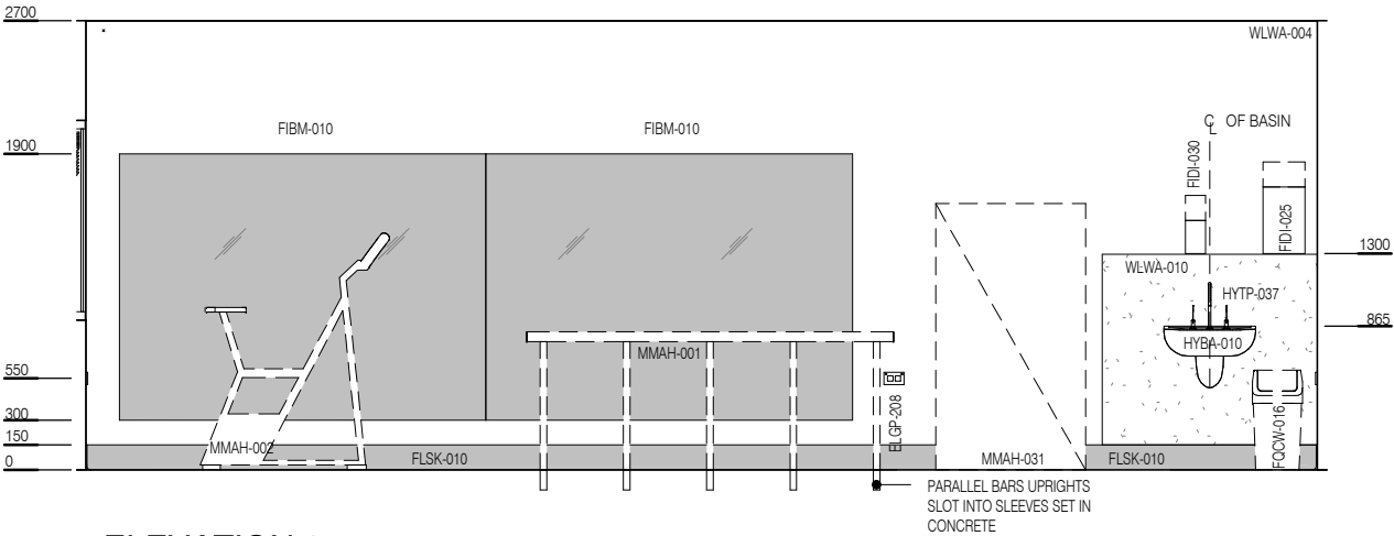
ELEVATION 2
