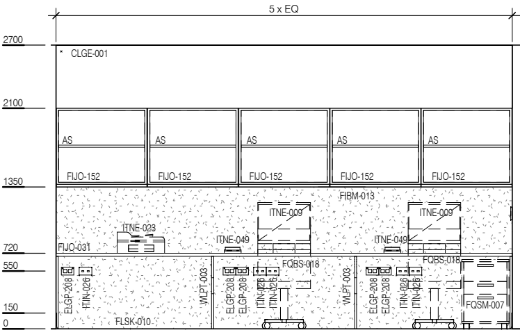
ELEVATION 4
