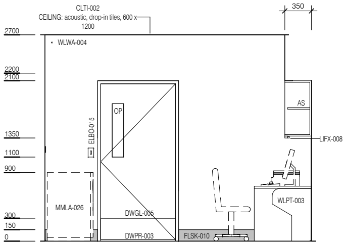
ELEVATION 3
