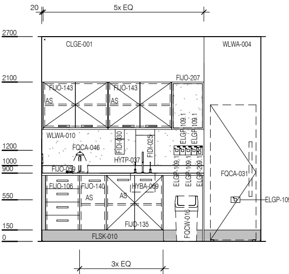
ELEVATION 4
