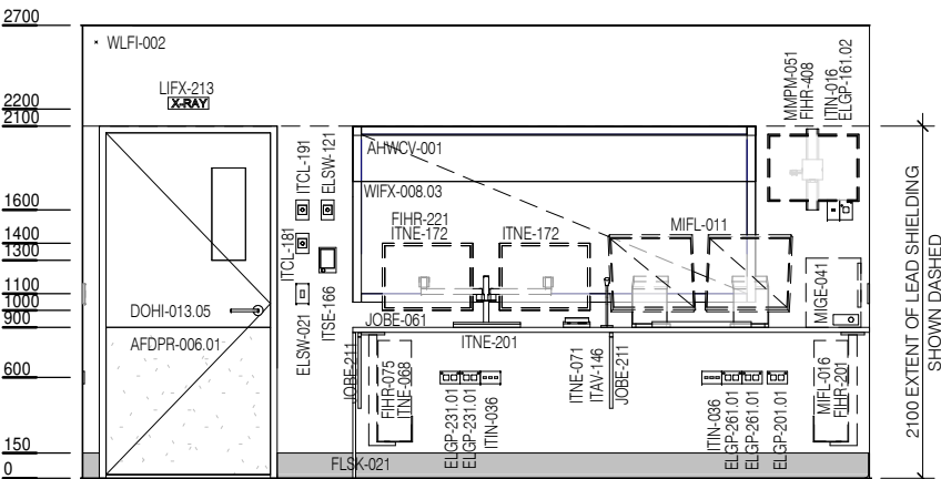
ELEVATION 2
