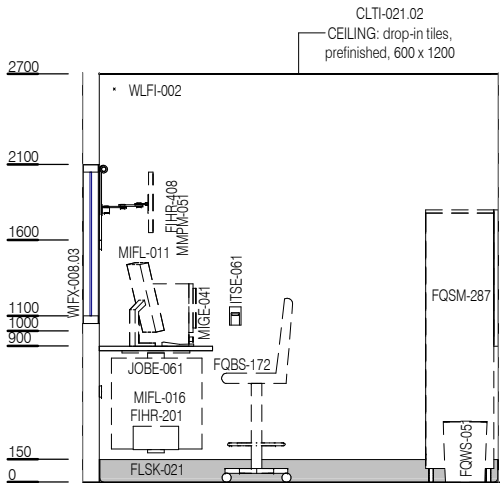
ELEVATION 3
