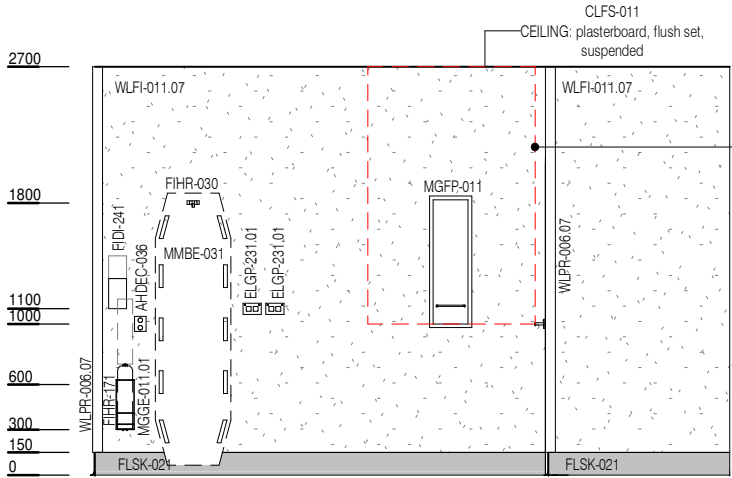
ELEVATION 1
