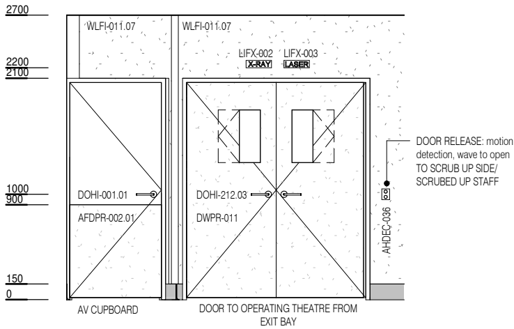
ELEVATION 2
