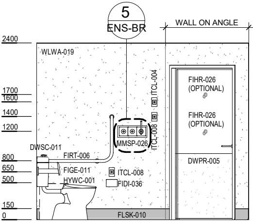
ELEVATION 4
