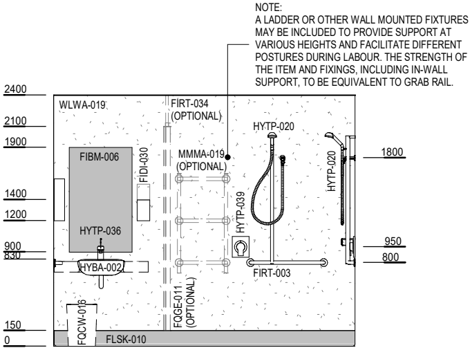
ELEVATION 2
