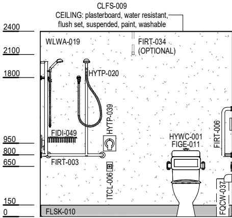
ELEVATION 3
