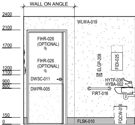
ELEVATION 1
