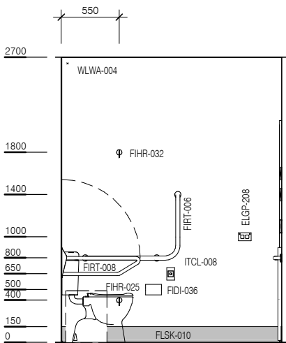
ELEVATION 4
