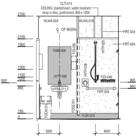
ELEVATION 2
