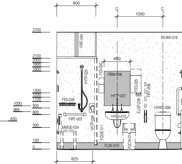
ELEVATION 4
