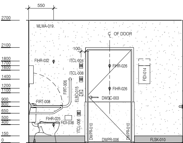
ELEVATION 1
