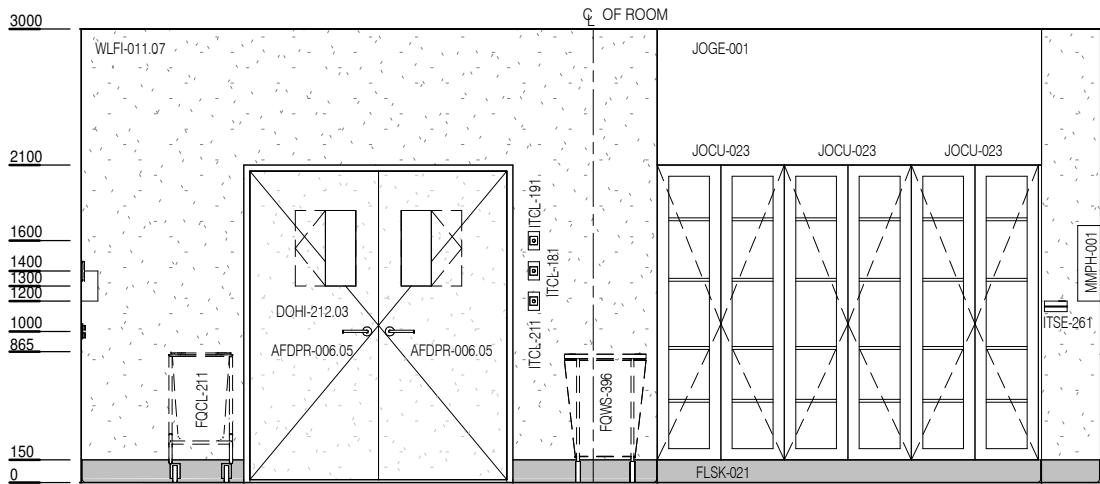
ELEVATION 3
