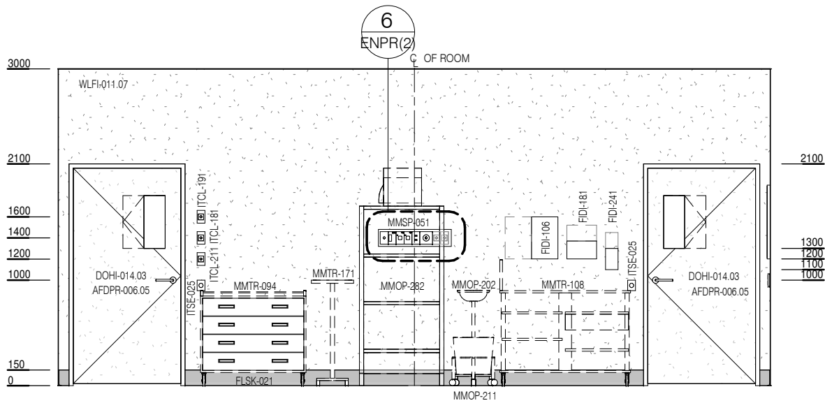
ELEVATION 1
