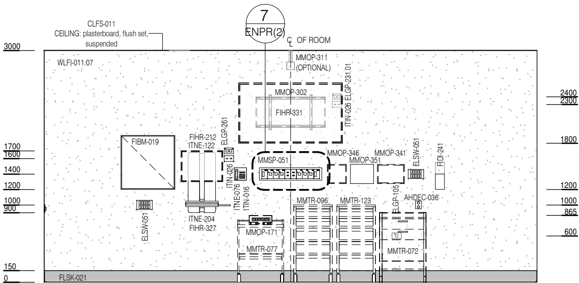
ELEVATION 2
