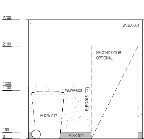
ELEVATION 1
