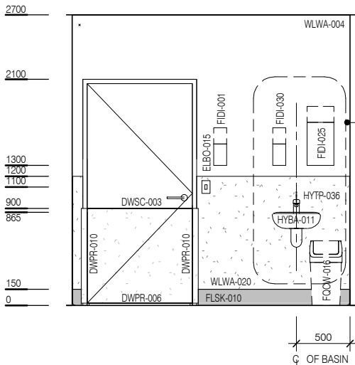
ELEVATION 3
