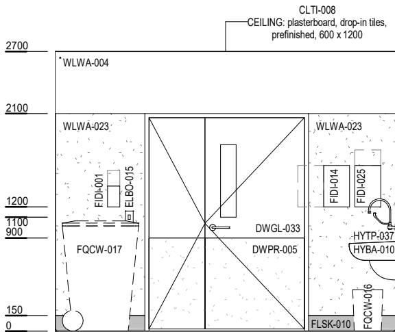
ELEVATION 3
