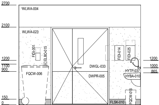
ELEVATION 3
