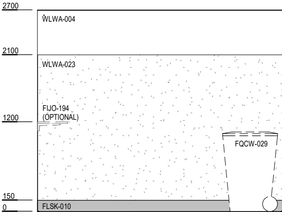
ELEVATION 1
