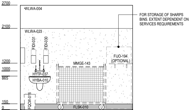
ELEVATION 4
