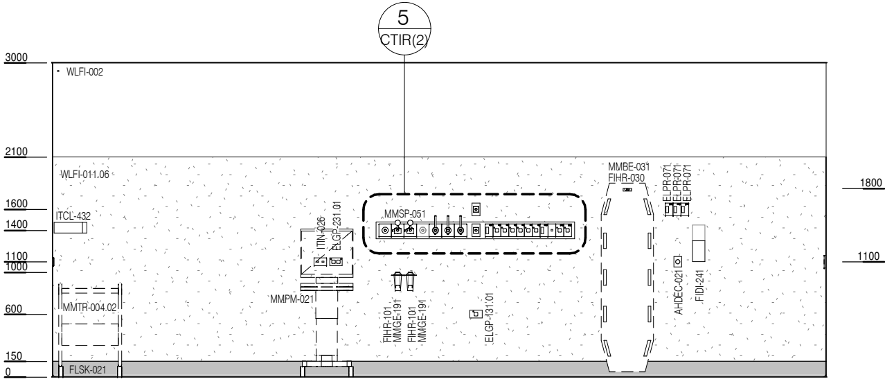
ELEVATION 2
