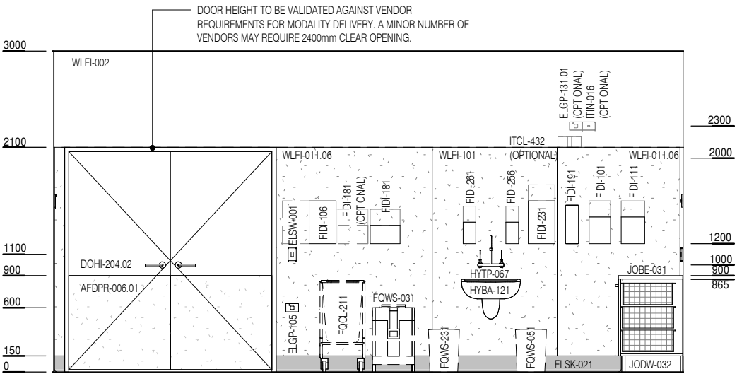
ELEVATION 3
