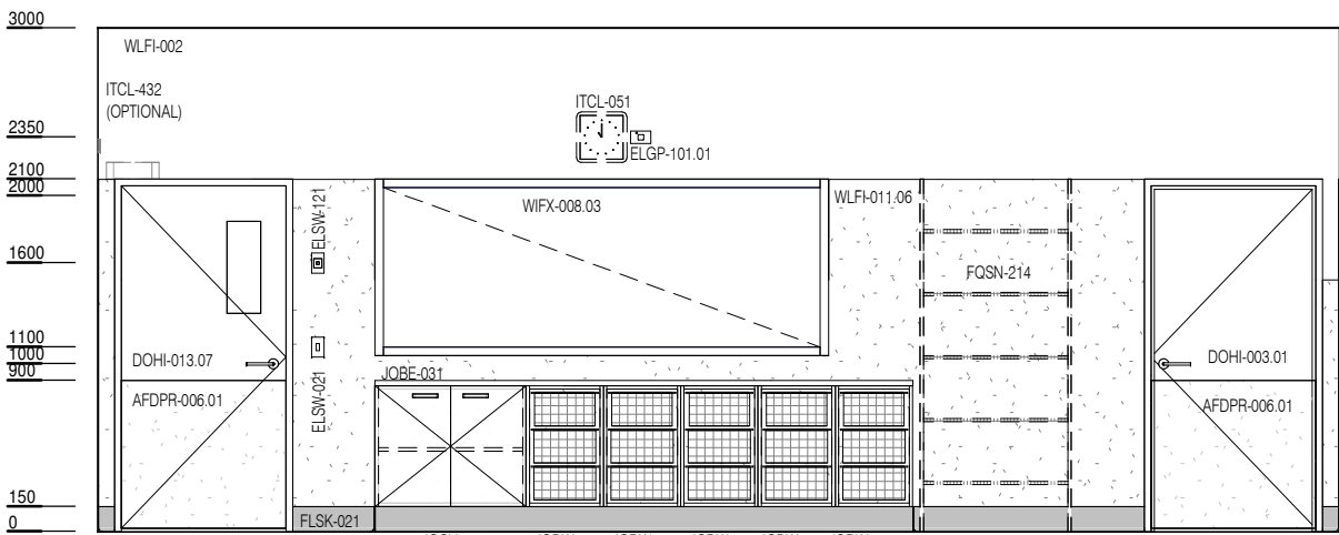
ELEVATION 4
