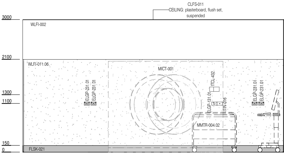
ELEVATION 1
