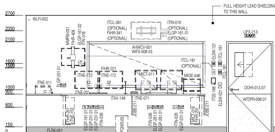
ELEVATION 2
