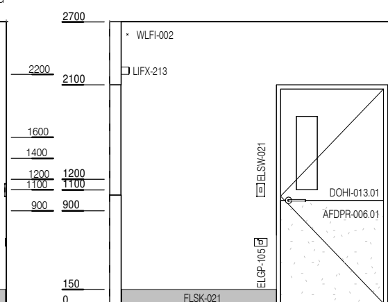
ELEVATION 3
