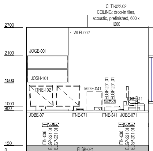
ELEVATION 1
