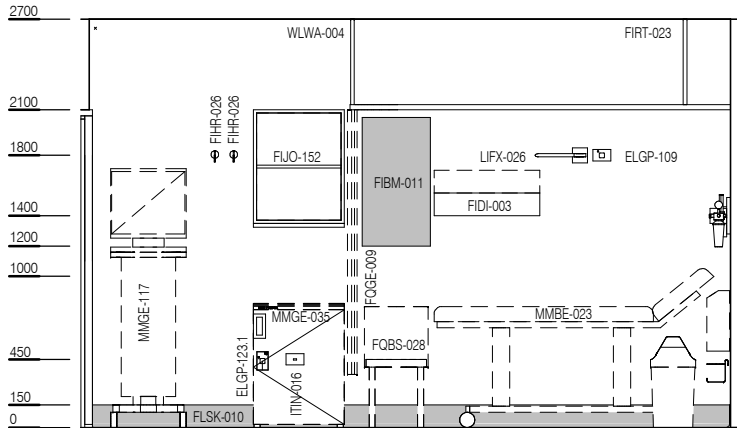
ELEVATION 4
