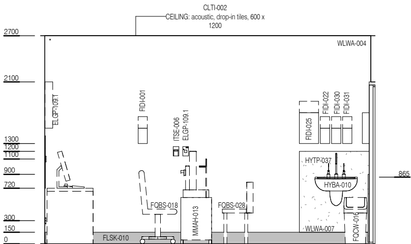
ELEVATION 2
