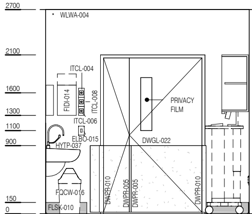
ELEVATION 3
