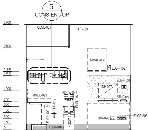
ELEVATION 1
