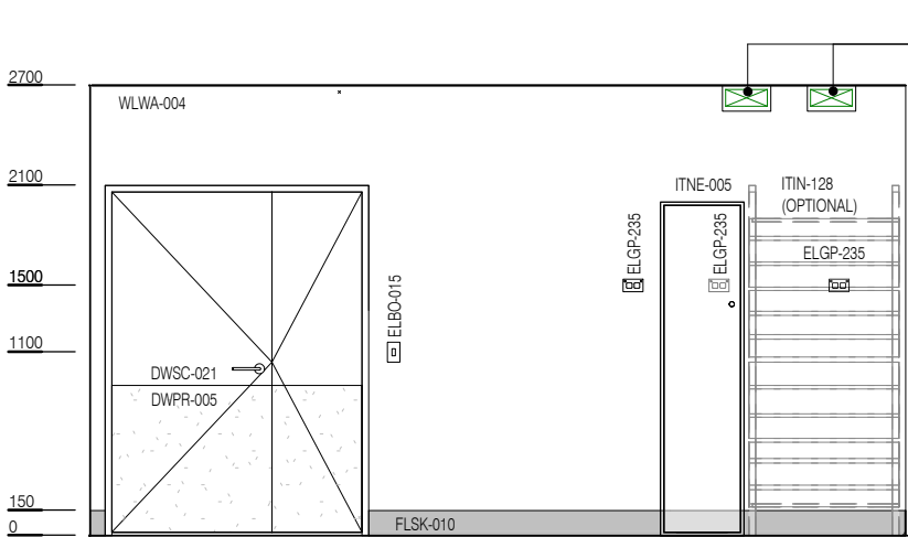
ELEVATION 3
