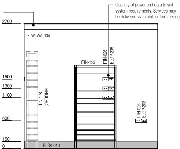
ELEVATION 4
