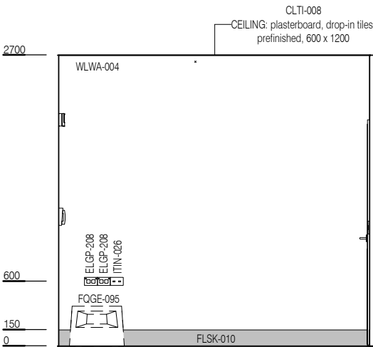
ELEVATION 2
