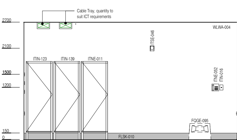
ELEVATION 1
