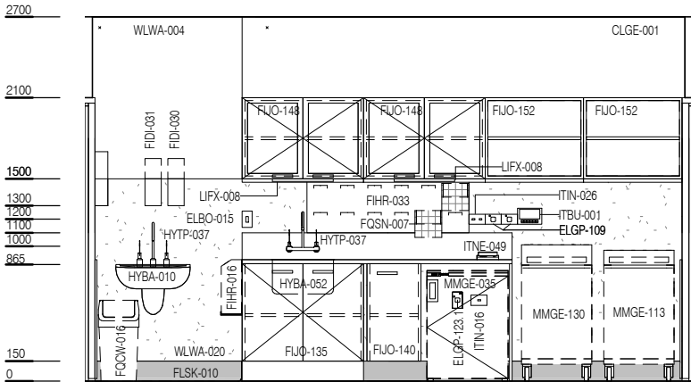
ELEVATION 4
