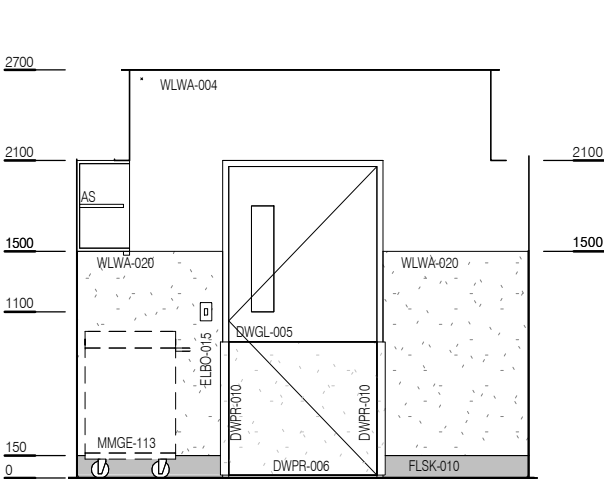
ELEVATION 1
