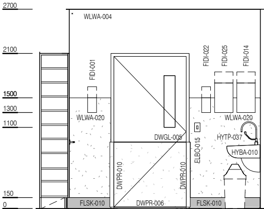
ELEVATION 3
