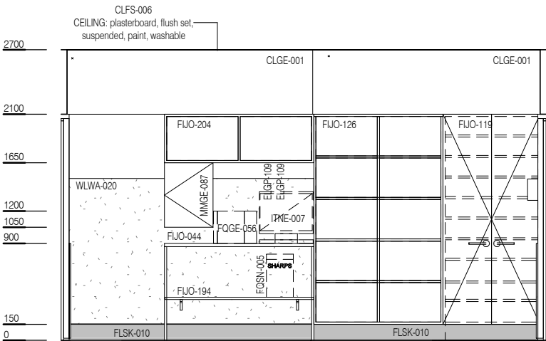
ELEVATION 2
