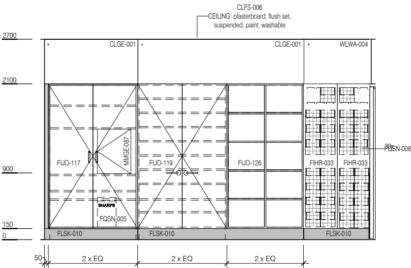
ELEVATION 1
