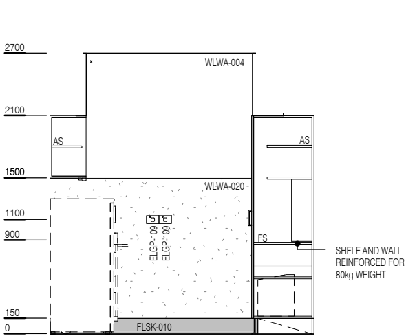
ELEVATION 1
