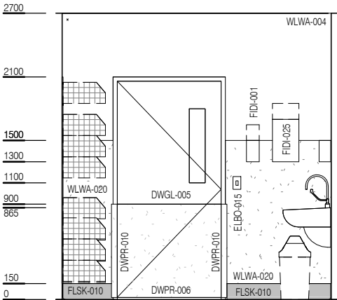
ELEVATION 3
