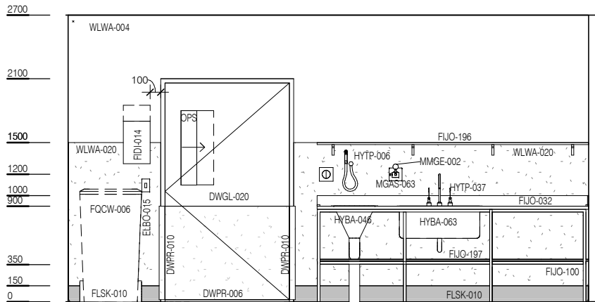
ELEVATION 4
