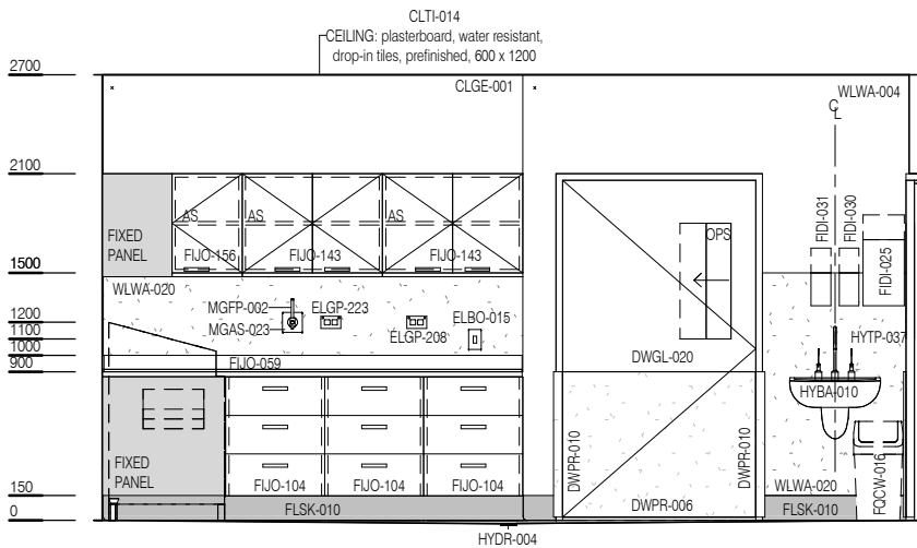
ELEVATION 2
