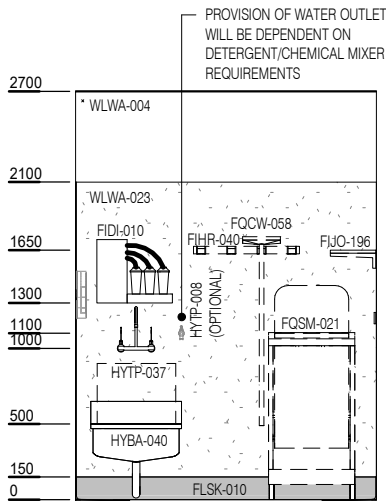
ELEVATION 1
