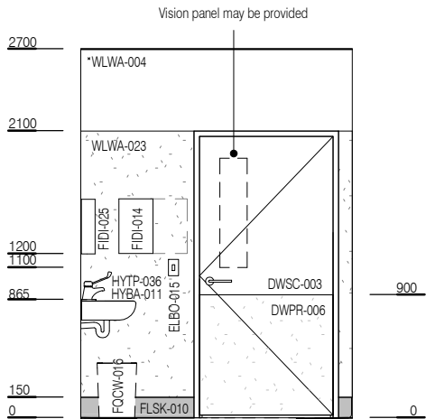
ELEVATION 3
