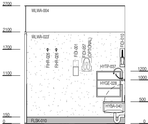
ELEVATION 4
