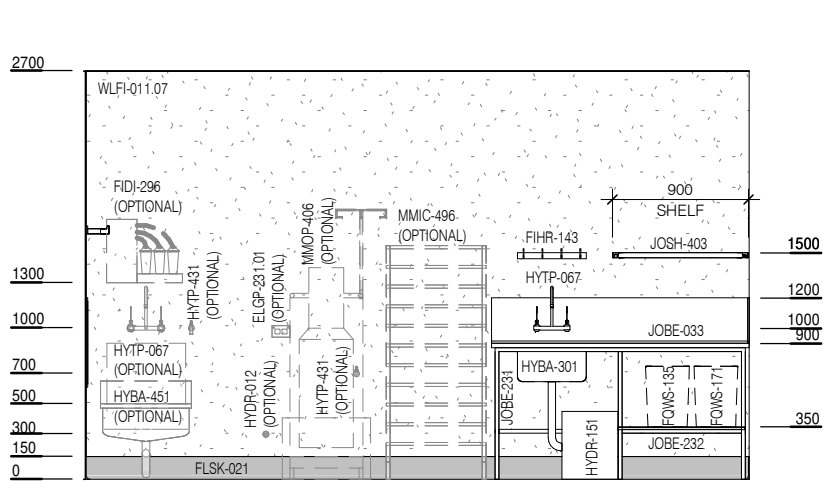
ELEVATION 1
