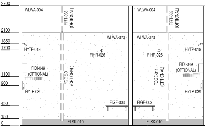
ELEVATION 1
