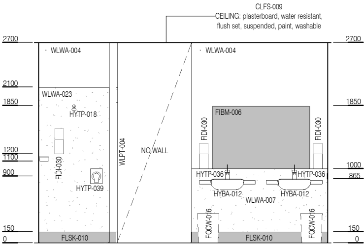
ELEVATION 2
