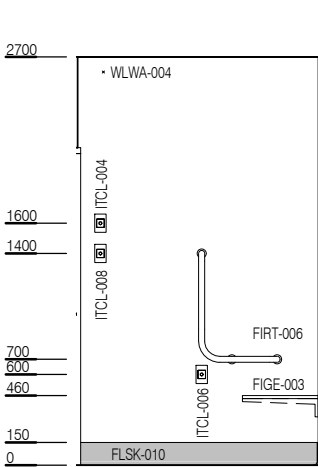
ELEVATION 1
