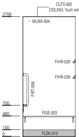
ELEVATION 2
