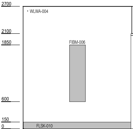
ELEVATION 3
