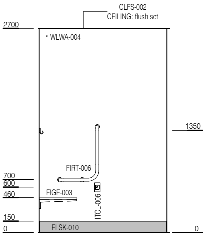
ELEVATION 2
