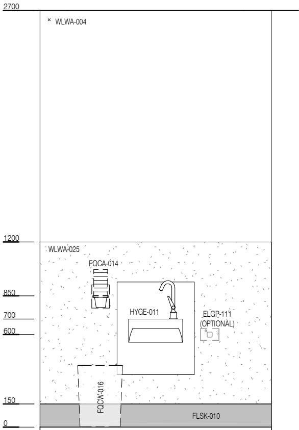
ELEVATION 2
