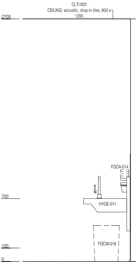
ELEVATION 1
