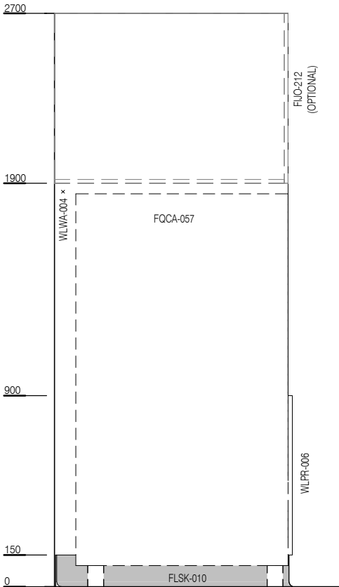
ELEVATION 3
