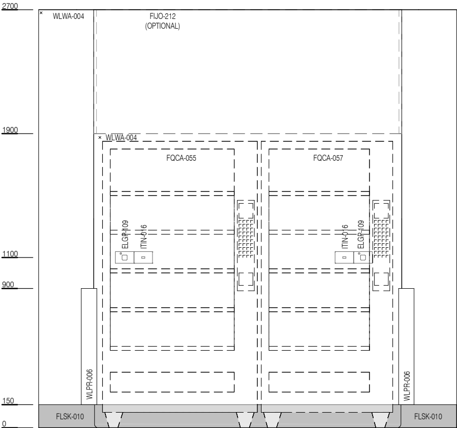
ELEVATION 2
