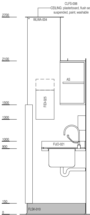
ELEVATION 1
