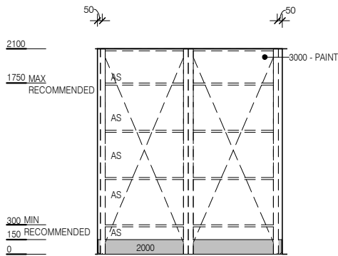
ELEVATION 2
