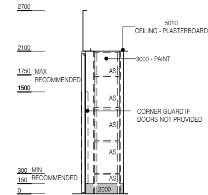
ELEVATION 1
