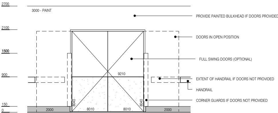
ELEVATION 3
