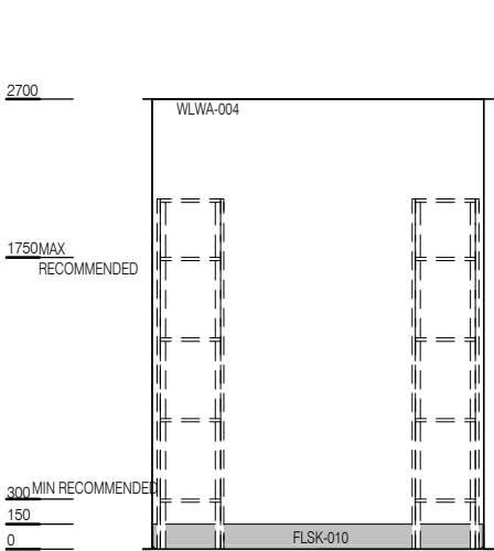
ELEVATION 1
