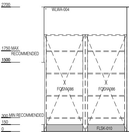
ELEVATION 4
