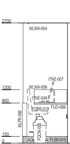
ELEVATION 1
