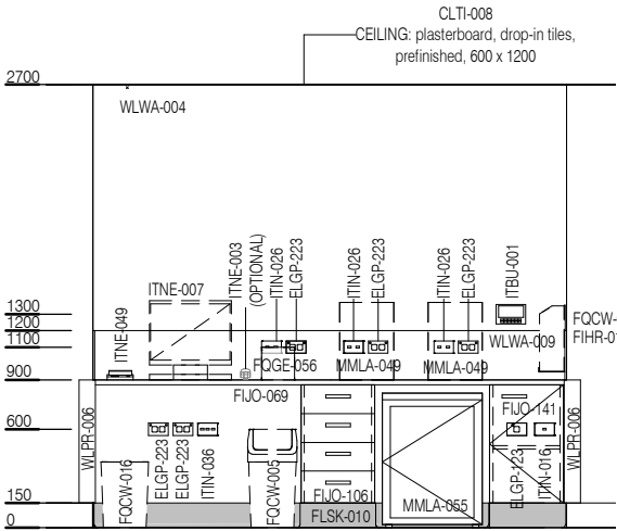
ELEVATION 2
