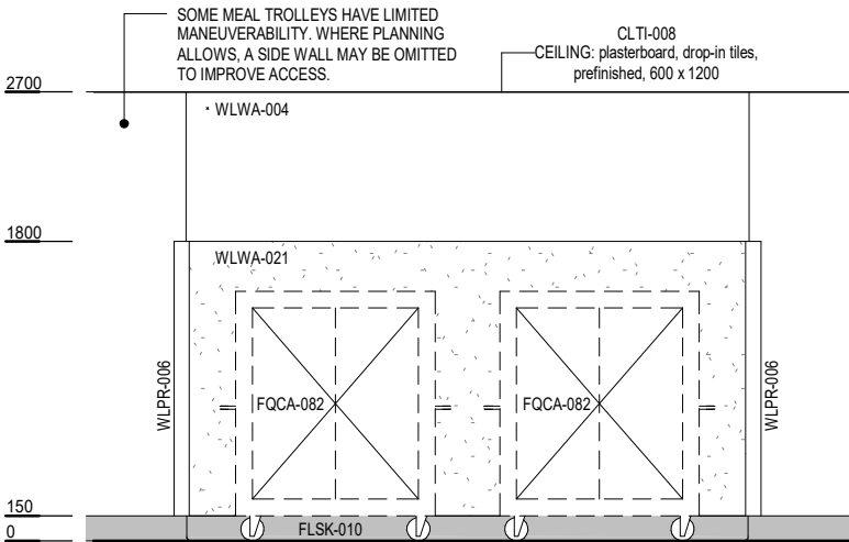
ELEVATION 2
