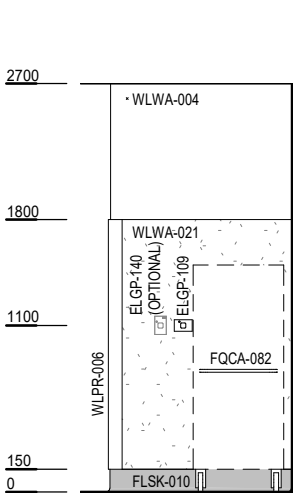
ELEVATION 1
