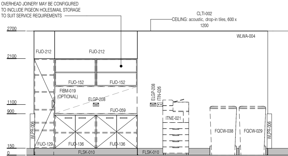
ELEVATION 2
