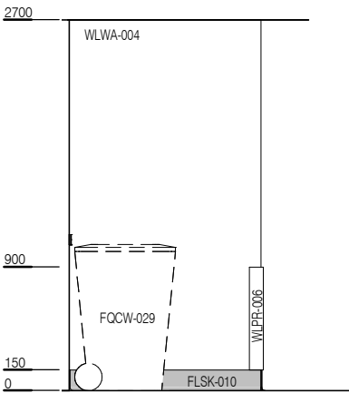
ELEVATION 3
