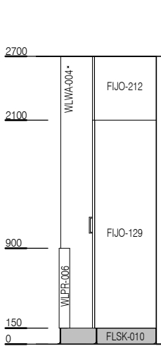
ELEVATION 1
