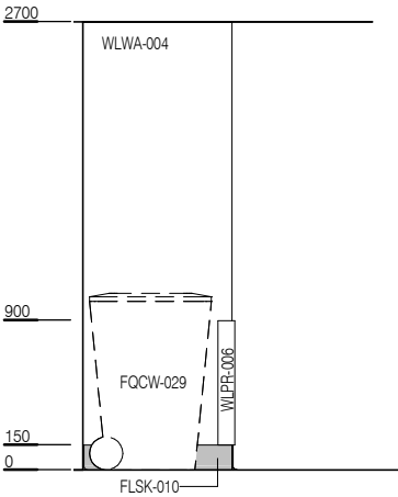
ELEVATION 3
