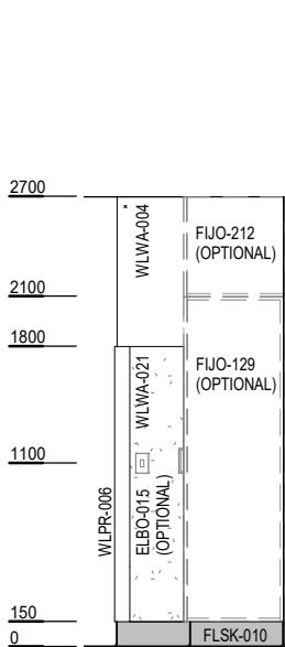
ELEVATION 1
