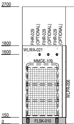
ELEVATION 3
