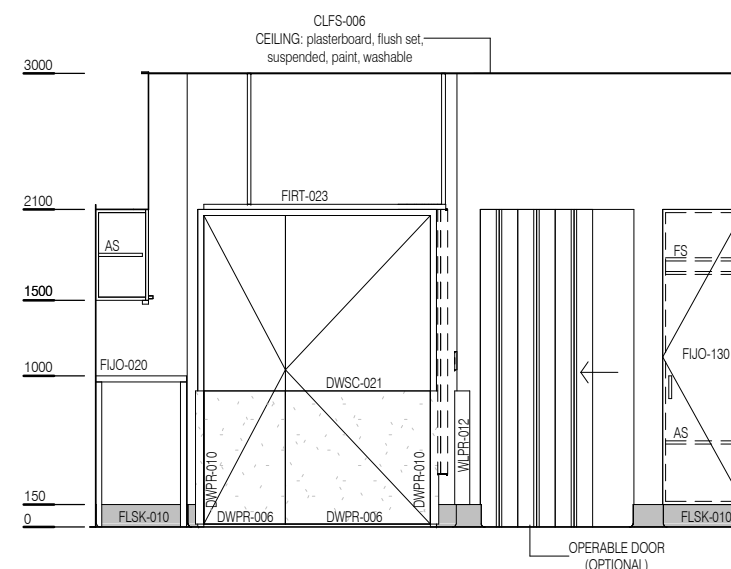
ELEVATION 4
