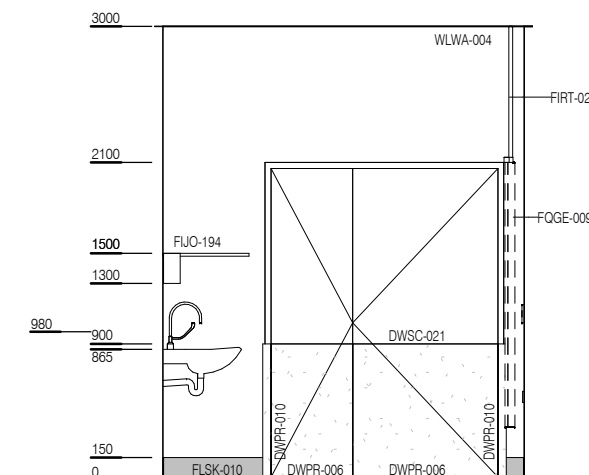
ELEVATION 5
