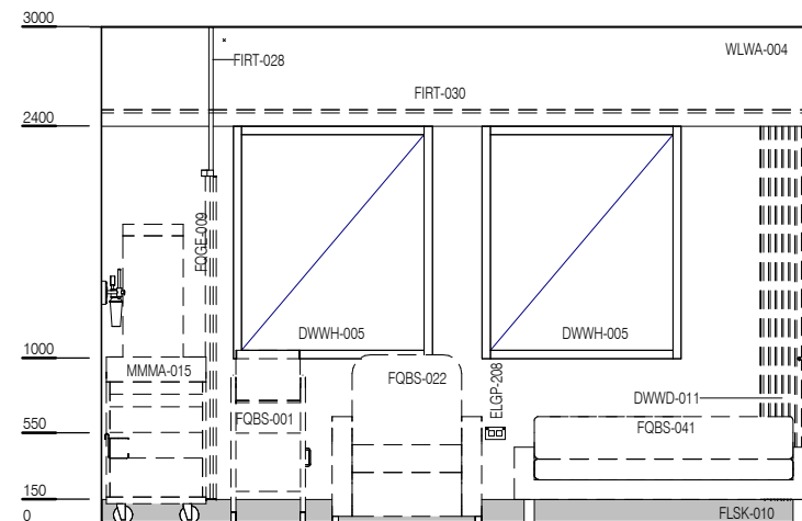
ELEVATION 2
