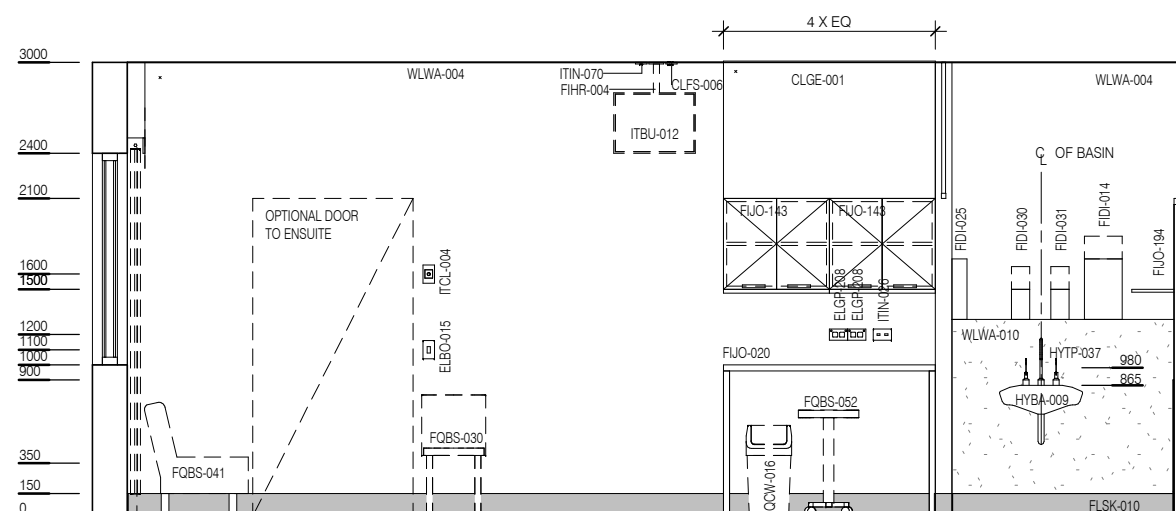
ELEVATION 3
