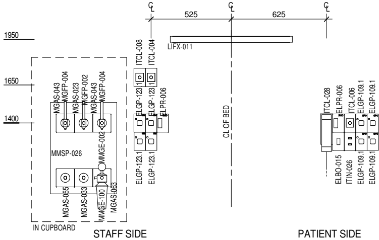
ELEVATION 5
