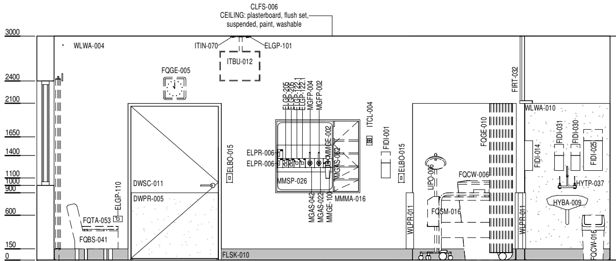
ELEVATION 1
