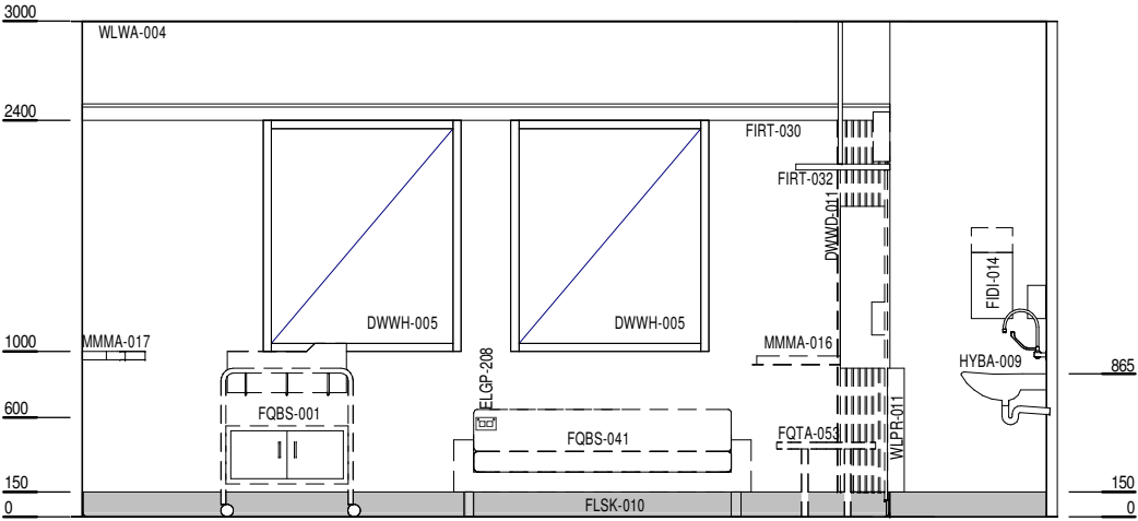
ELEVATION 2
