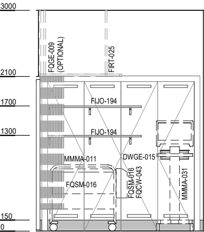
ELEVATION 6
