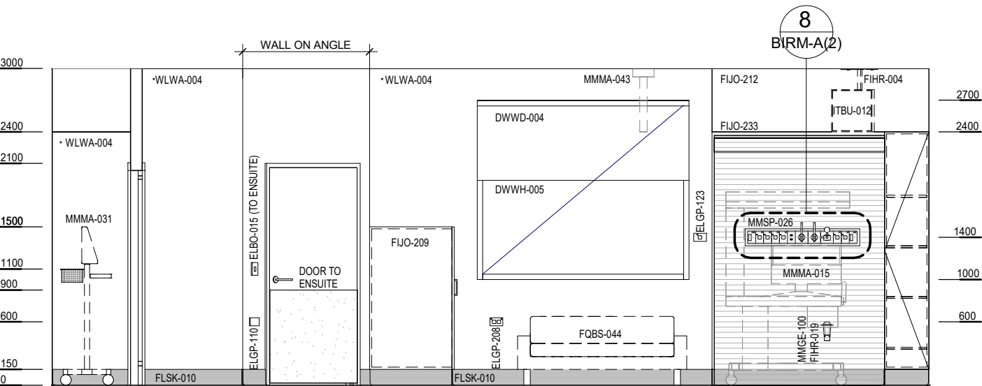
ELEVATION 1
