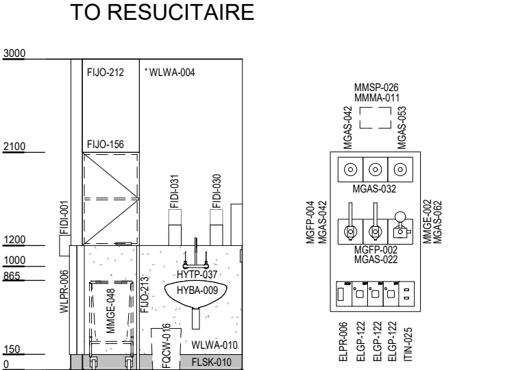
ELEVATION 5
