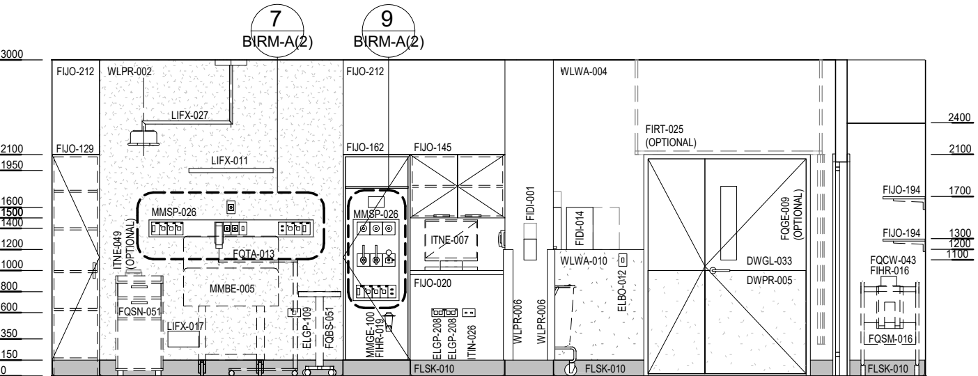
ELEVATION 3
