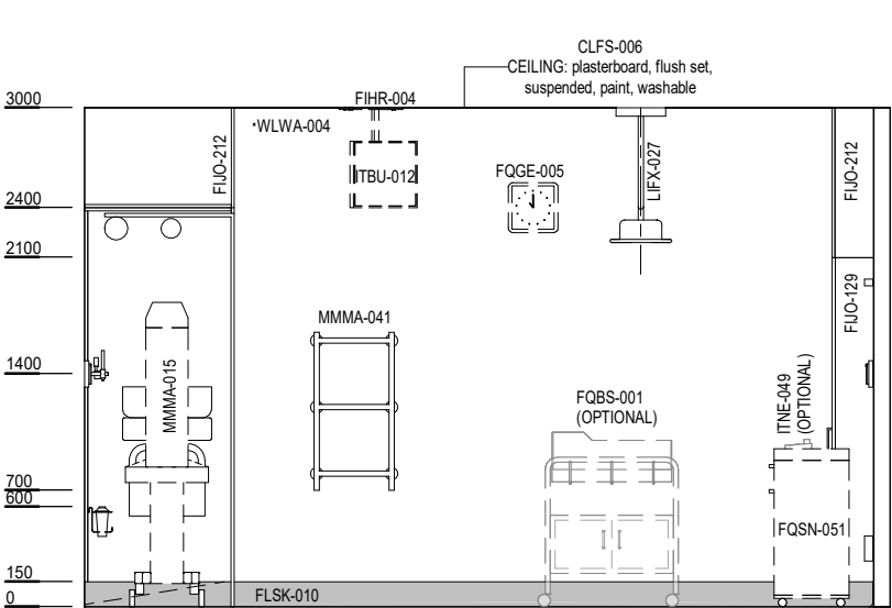
ELEVATION 2
