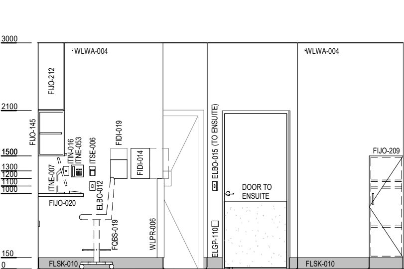
ELEVATION 4
