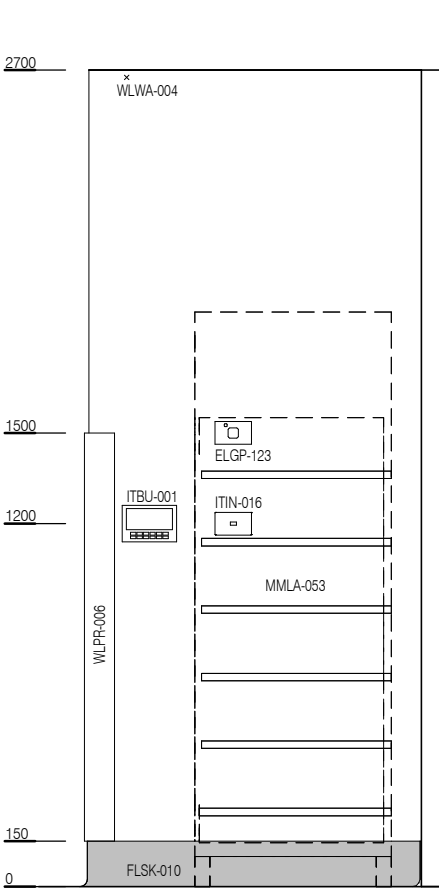
ELEVATION 1
