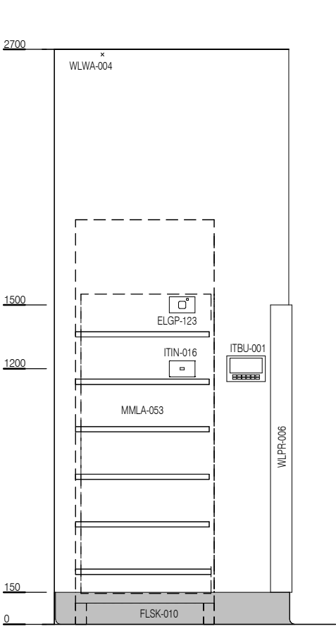
ELEVATION 3
