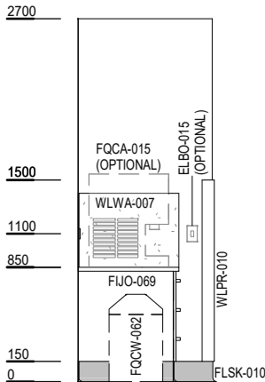
ELEVATION 3
