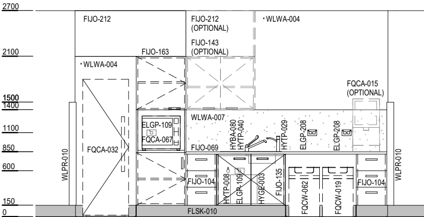
ELEVATION 2
