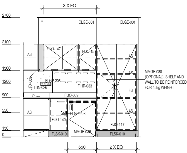
ELEVATION 1
