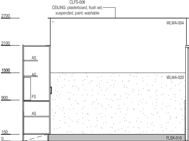
ELEVATION 2
