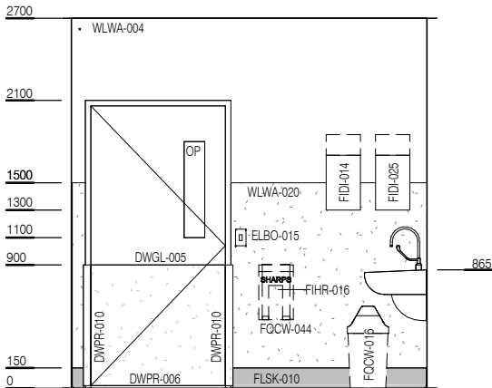
ELEVATION 3
