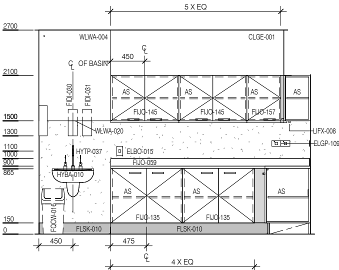
ELEVATION 4
