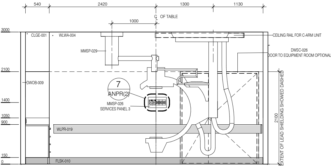
ELEVATION 1
