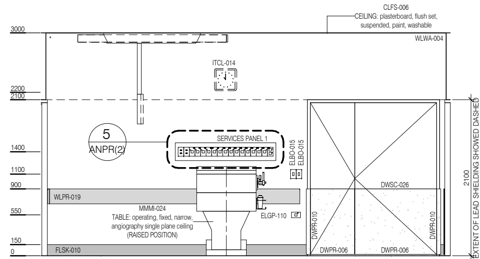
ELEVATION 3
