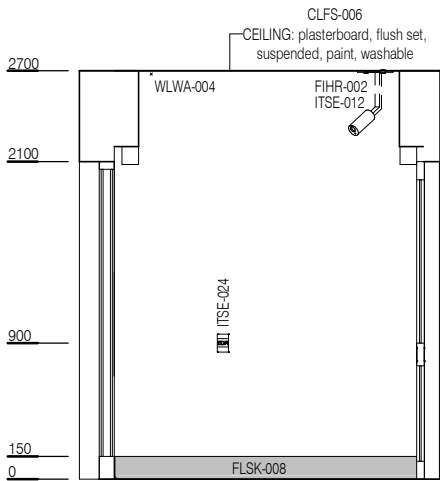
ELEVATION 5
