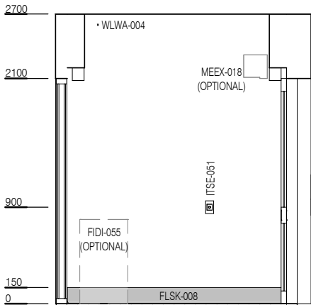
ELEVATION 4
