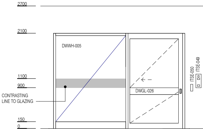
ELEVATION 5
