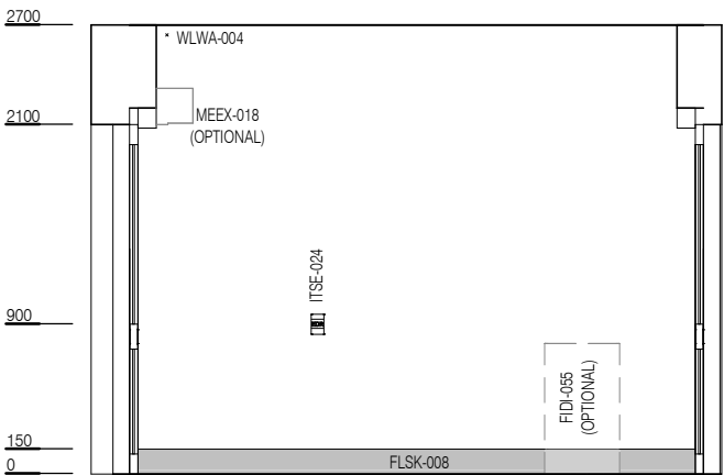
ELEVATION 2
