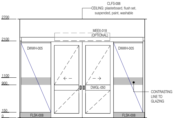
ELEVATION 1
