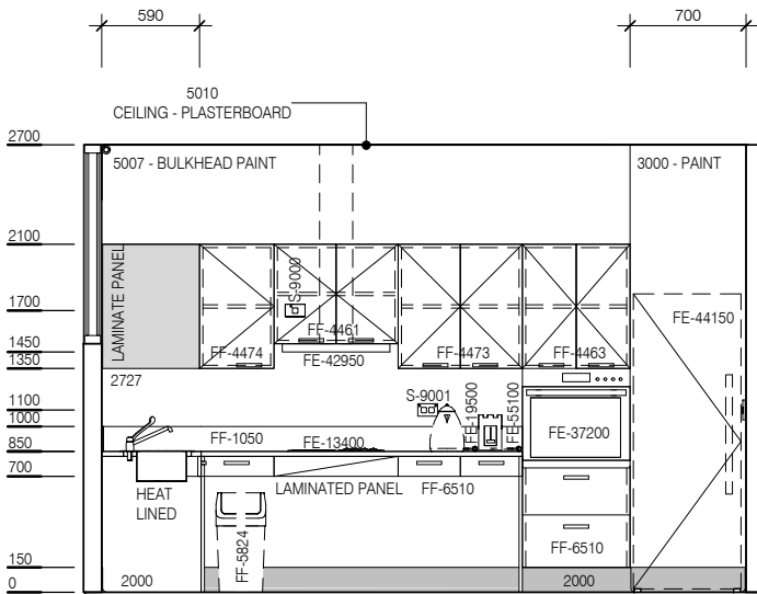
ELEVATION 2
