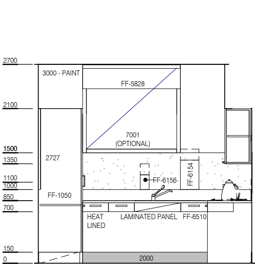
ELEVATION 1
