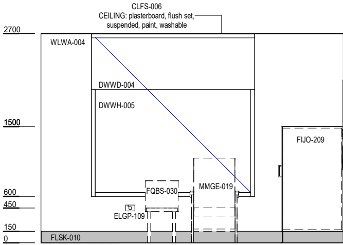
ELEVATION 1
