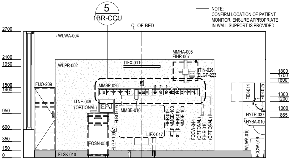
ELEVATION 2
