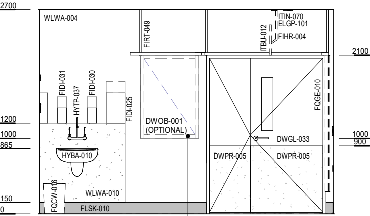
ELEVATION 3
