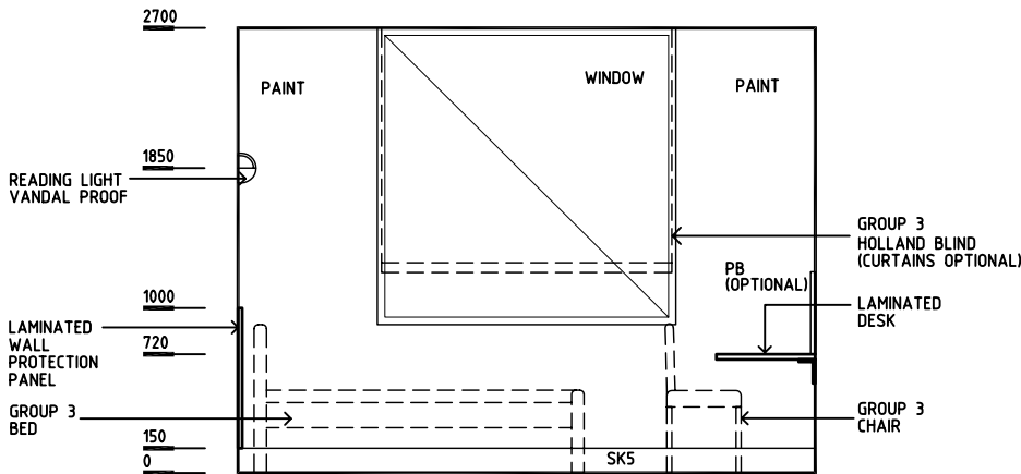
ELEVATION 1
