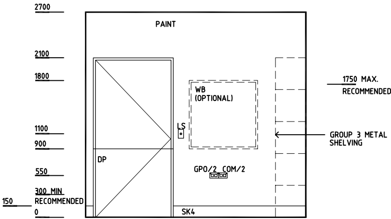
ELEVATION 3
